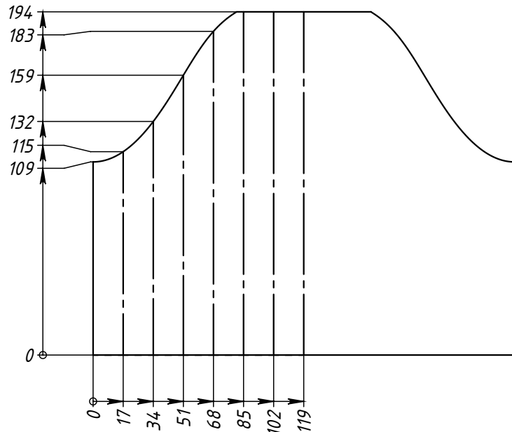
Поз.2 (Труба) развертка
